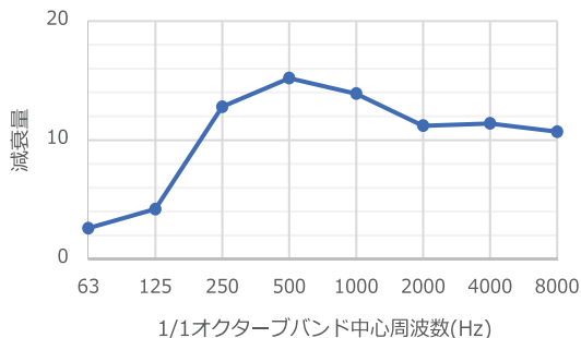
[サイレンサーの減音効果例]
